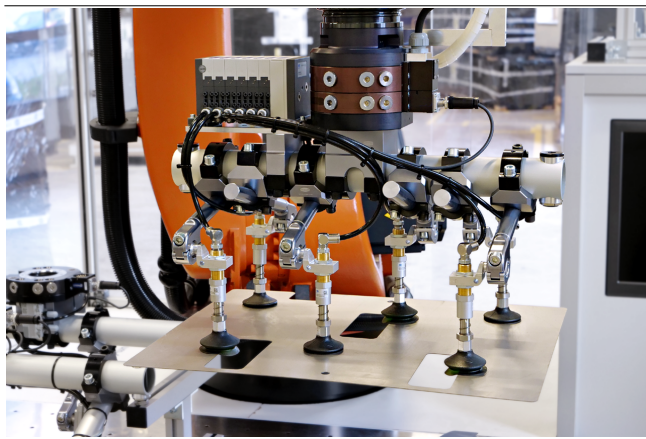
Зажимные элементы с удлинителем SXT-CL-EXT в сочетании с магнитными захватами SGM-HP при работе с формованной деталью из
